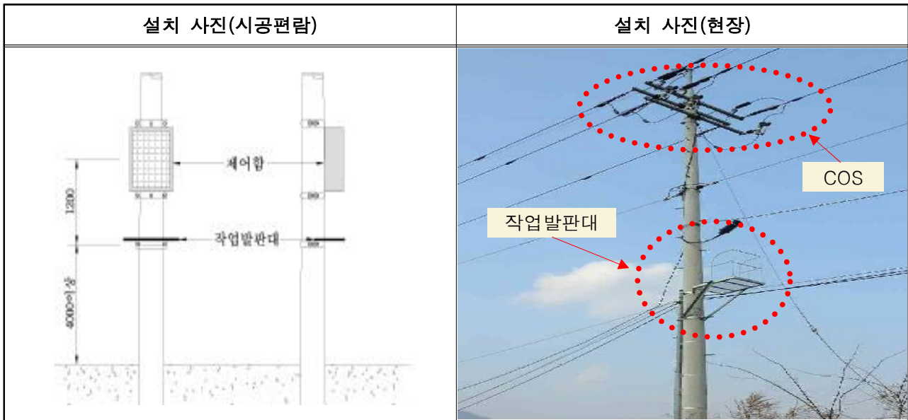
[그림 1] 작업발판대 설치 사진
